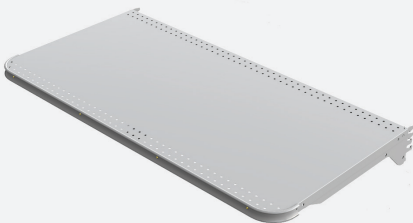
ITEM TABLETTE COINS RONDS FORMAT 24"- 30"- 36"- 48" (LONGUEUR) PROFONDEUR 16" À 24" (PAR INCRÉMENT DE 2")
