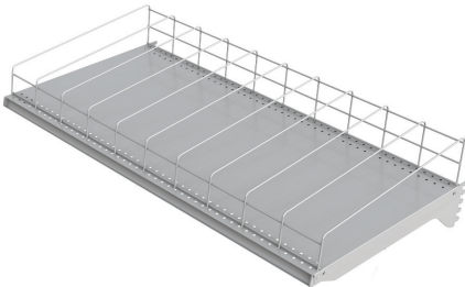
ITEM TABLETTE "LIQUEUR" FORMAT 24"- 30"- 36"- 48" (LONGUEUR) PROFONDEUR 6" À 30" (PAR INCRÉMENT DE 2")
