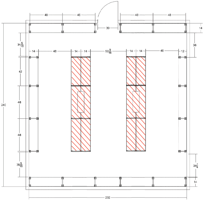
100 PIED LINÉAIRE D'ENTREPOSAGE PLAN DE PLANCHER AVEC UNITÉS FIXES
