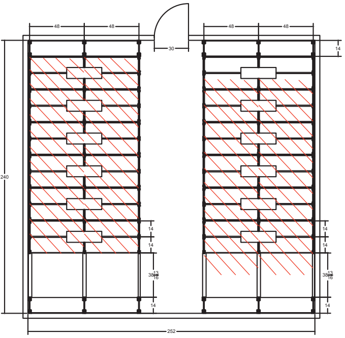
224 PIED LINÉAIRE D'ENTREPOSAGE PLAN DE PLANCHER AVEC UNITÉS MOBILES
