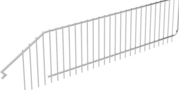
ITEM WIRE DIVIDER - 6" H FORMAT 10" - 12" - 14" - 16" - 18"
